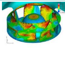
ファン流体騒音の解析
