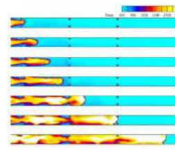
爆轟燃焼の解析
